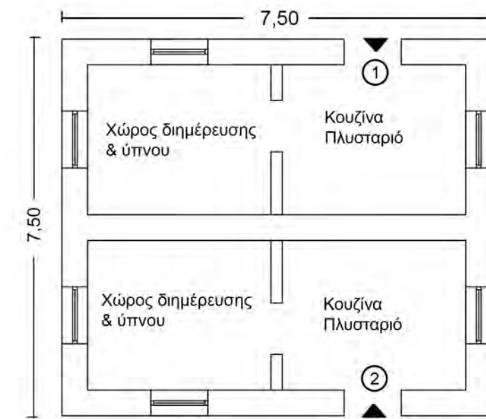
Κάτοψη
