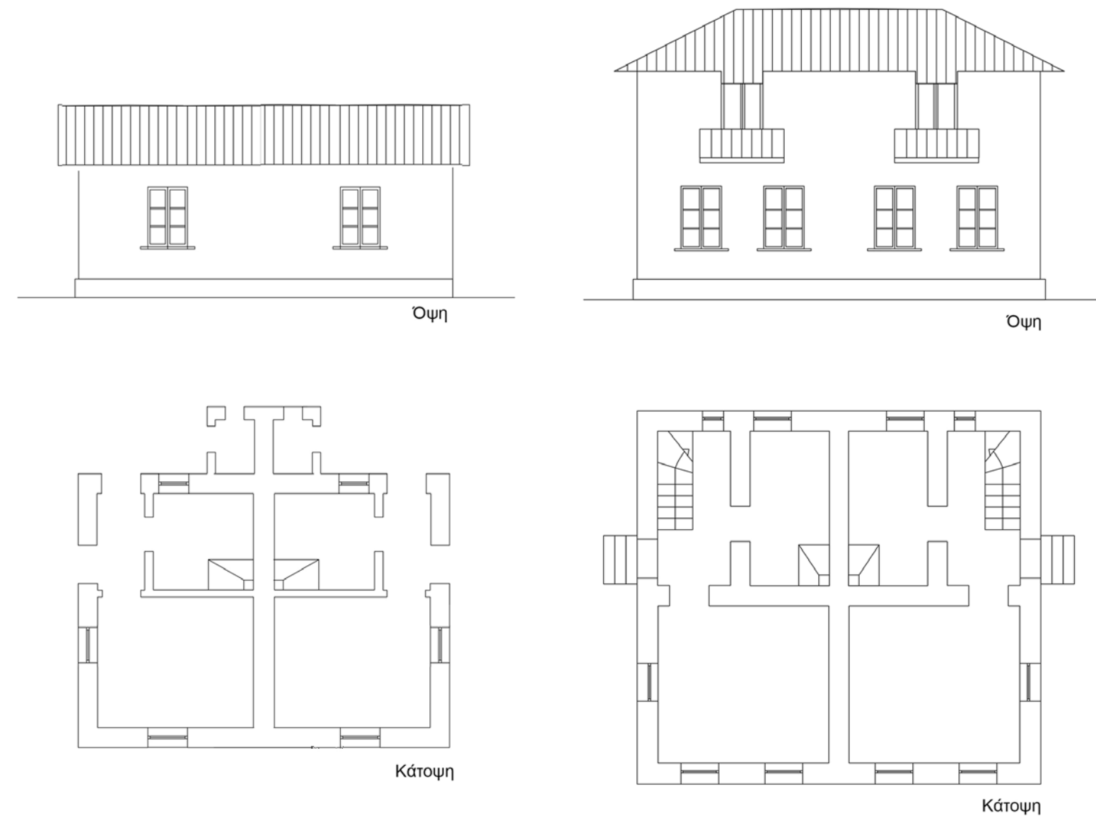
Εικ. 27 Τυπολογία ισόγειας και διώροφης αστικής προσφυγικής κατοικίας του Υπουργείου Πρόνοιας. Ψηφιακή επεξεργασία των πρωτότυπων σχεδίων από τη συγγραφέα. Βασιλείου 1944.
